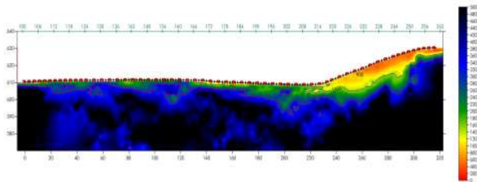
Sezione 2D da Tomografia in onde P
