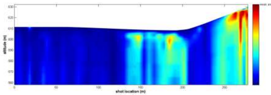
Sezione 2D da analisi della dispersione delle onde di superficie
