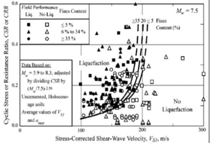
Depositi non cementati di età olocenica per M_w=7.5 (Andrus e Stokoe, 2000)
