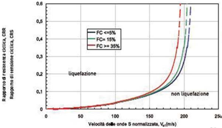
Depositi non cementati di età olocenica per M_w=7.5 (Andrus e Stokoe, 2000)
