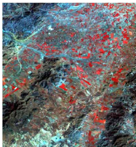
Valle di Guadalentín (Spagna) - Composite Landsat 421
